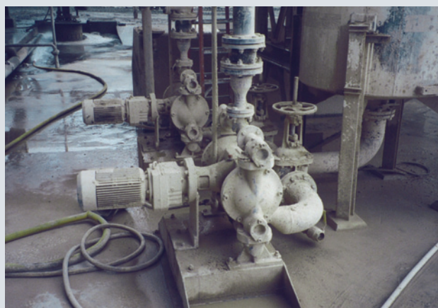
Pompes ABEL EM dans un dur fonctionnement continu
