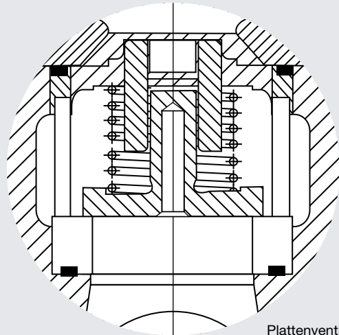
Plattenventil
