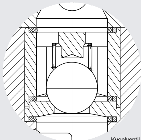
Kugelventil
