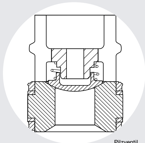
Pilzventil
